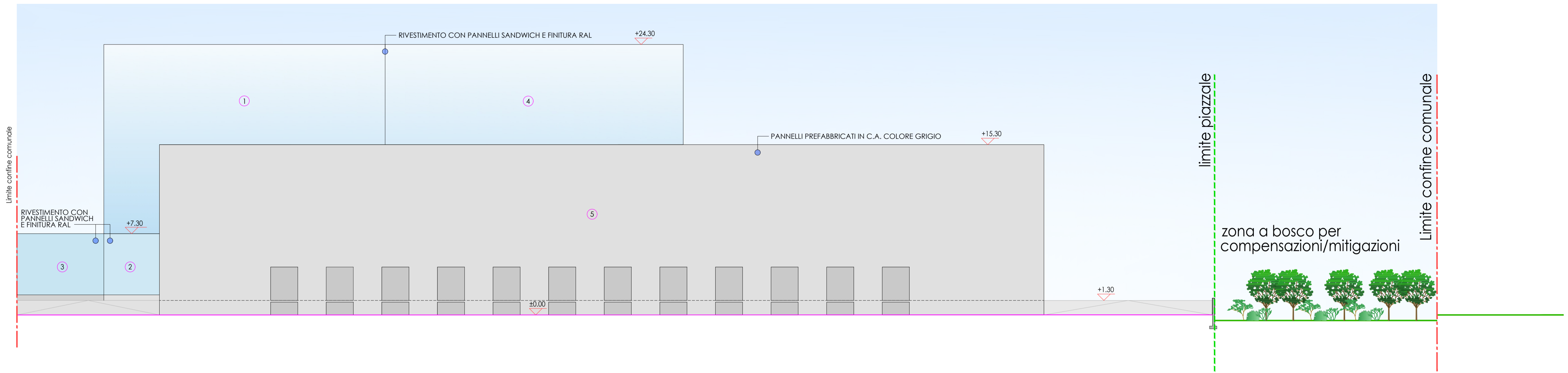
PROSPETTO NORD - stato di progetto scala 1:200
