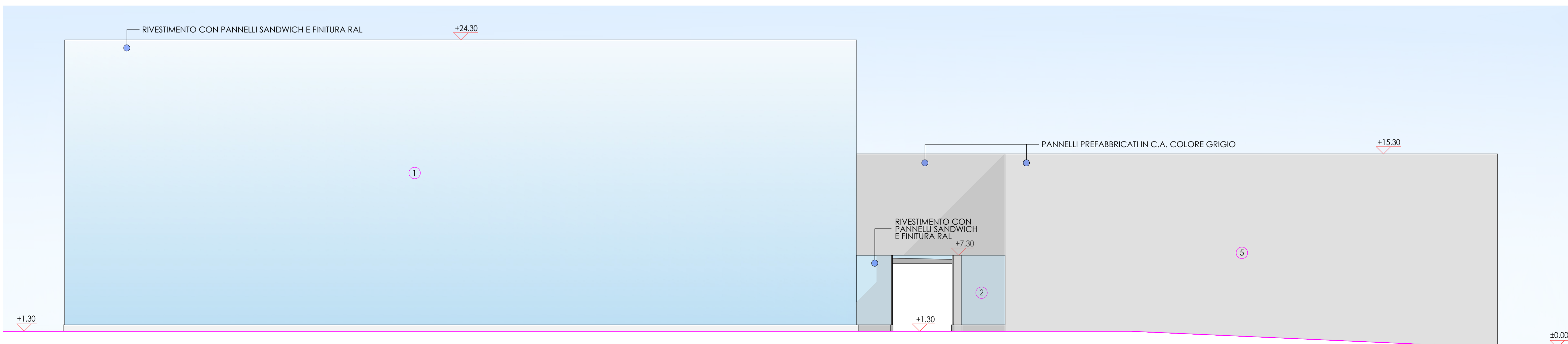
PROSPETTO OVEST - stato di progetto scala 1:200
