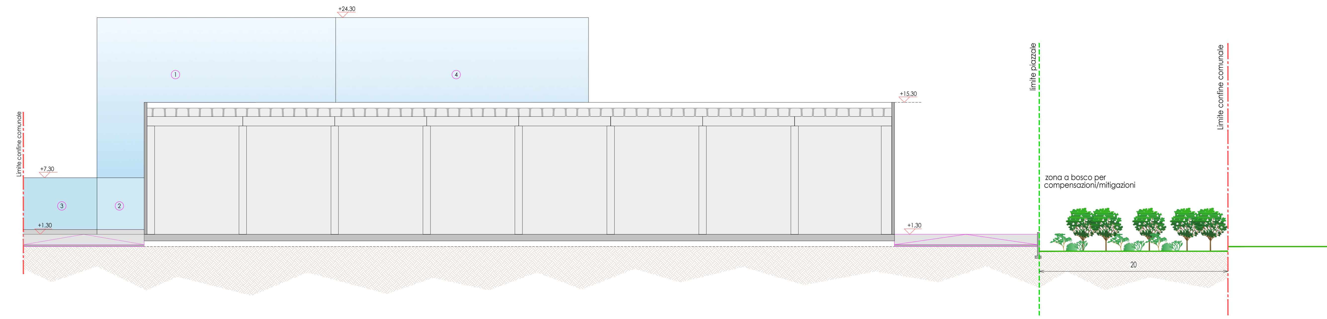
SEZIONE B-B - stato di progetto scala 1:500
