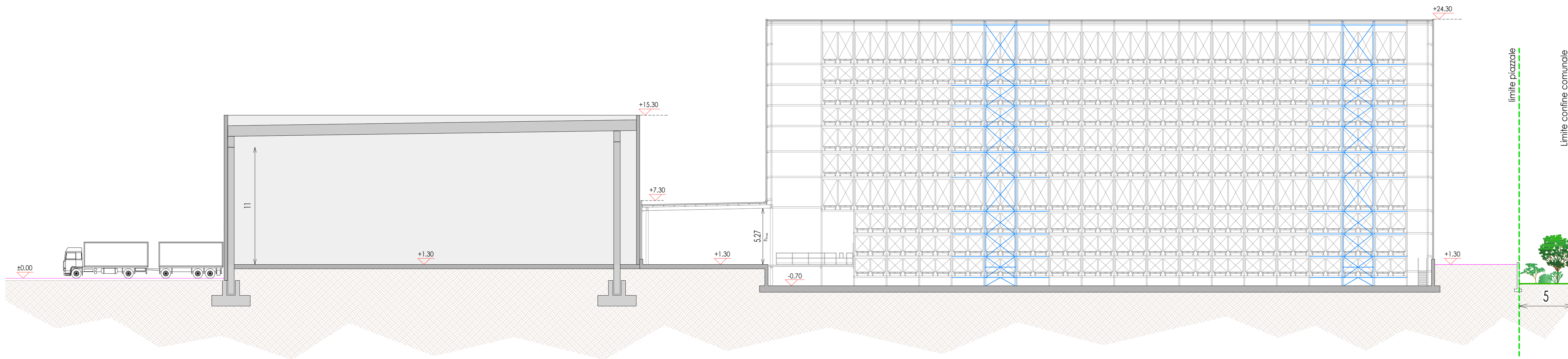
SEZIONE D-D - stato di progetto scala 1:500
